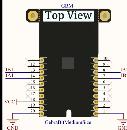
GEBRABIT PINOUT
